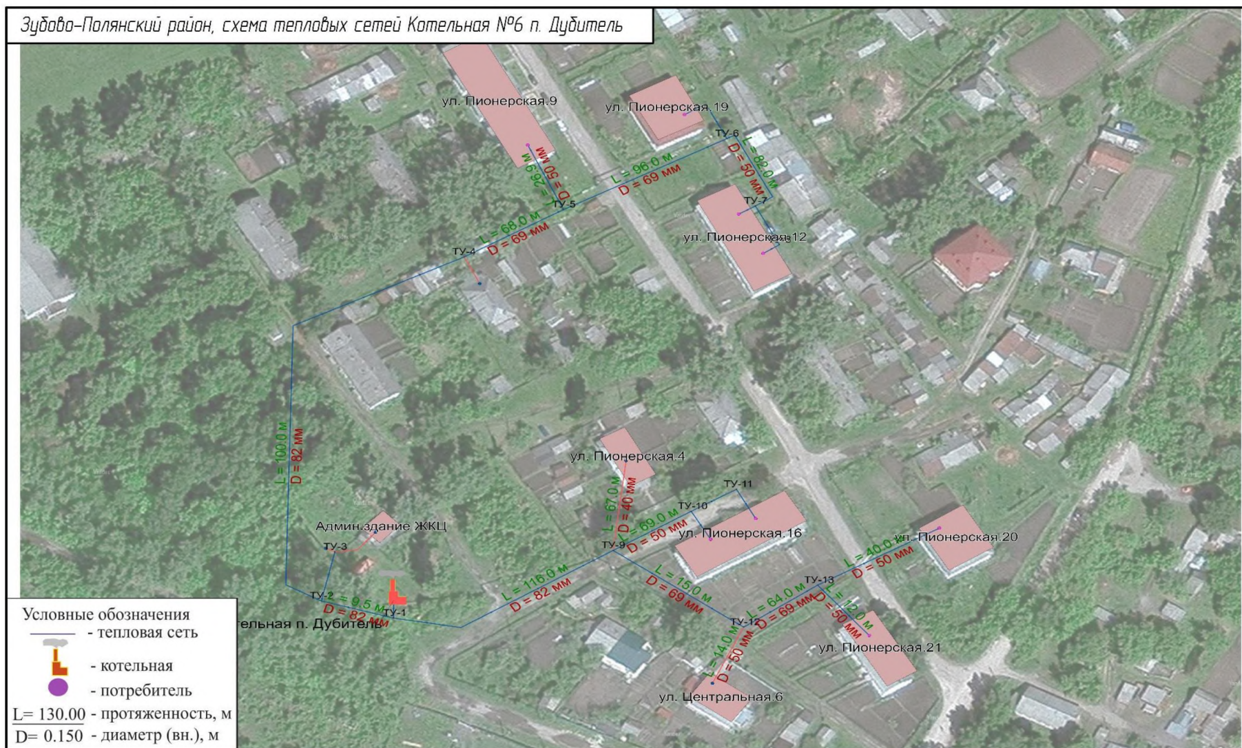
Рисунок 2. Зона действия котельной №6 п. Дубитель (МП Zubovo-Полянского муниципального района «Тепловые сети»)
